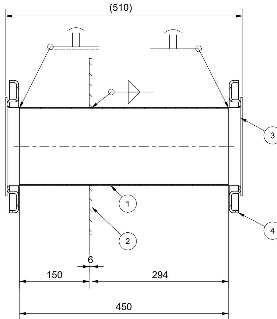
A-A ( 1 : 5 )
