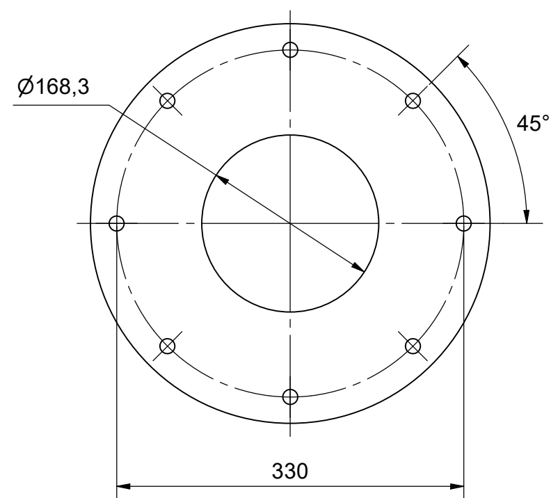
Sheet Plate ( 1 : 5 )
